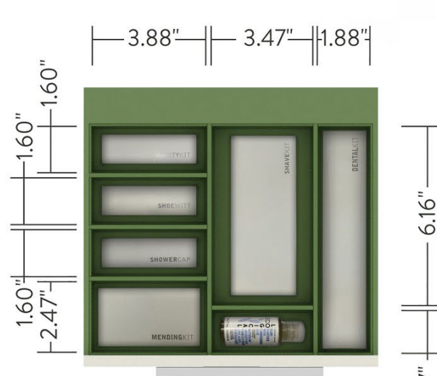
top elevation
